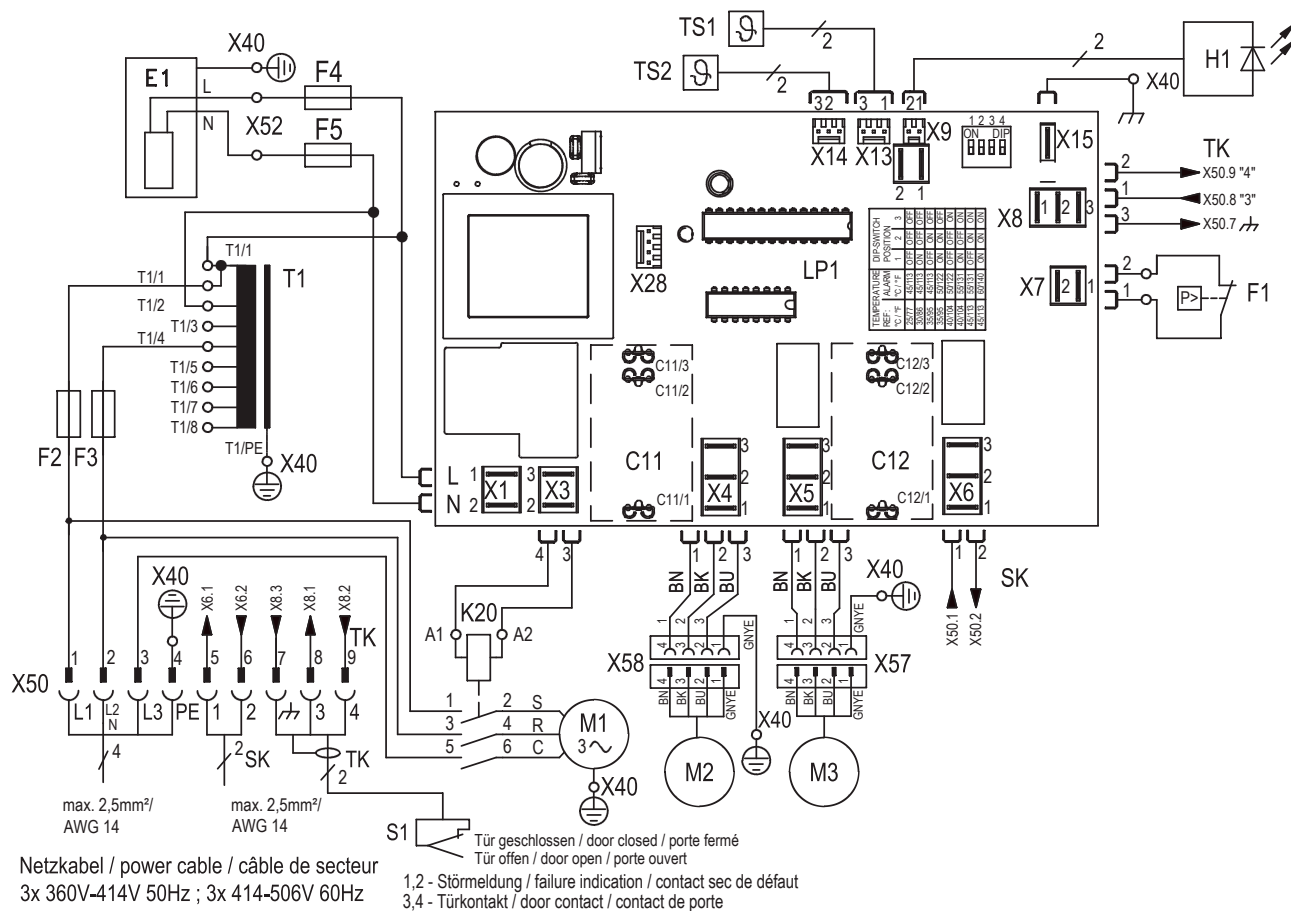
Рис. 20: Принципиальная электрическая схема
