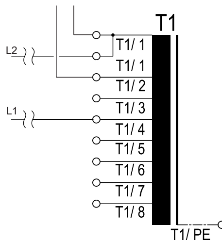
Eingangswicklung Steuertransformator
