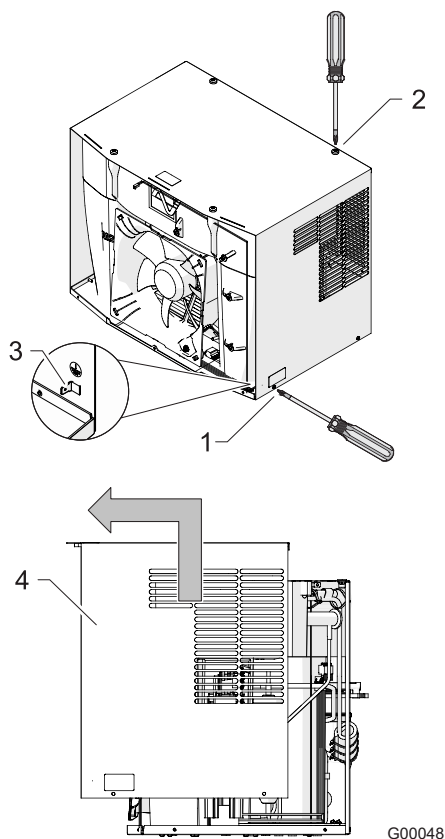
Рис. 28: Снятие передней панели
