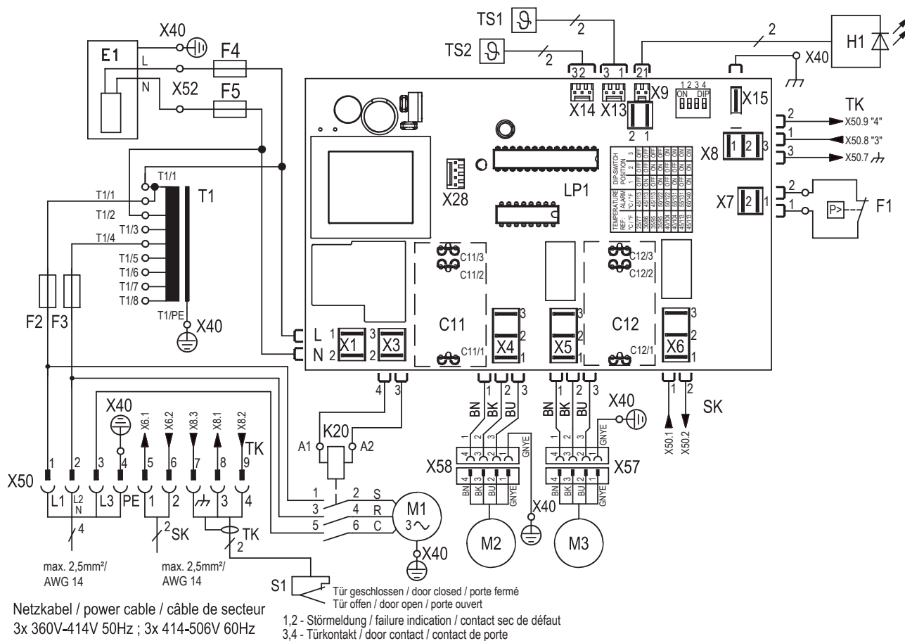
Fig. 20: Schema elettrico
