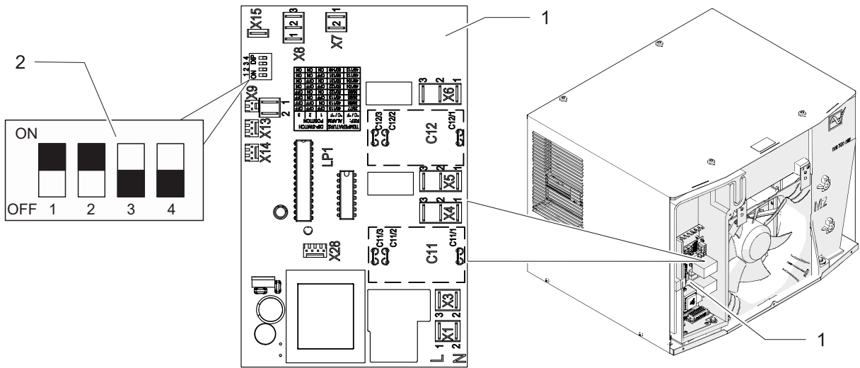
Рис. 21: Настройка DIP-переключателя
