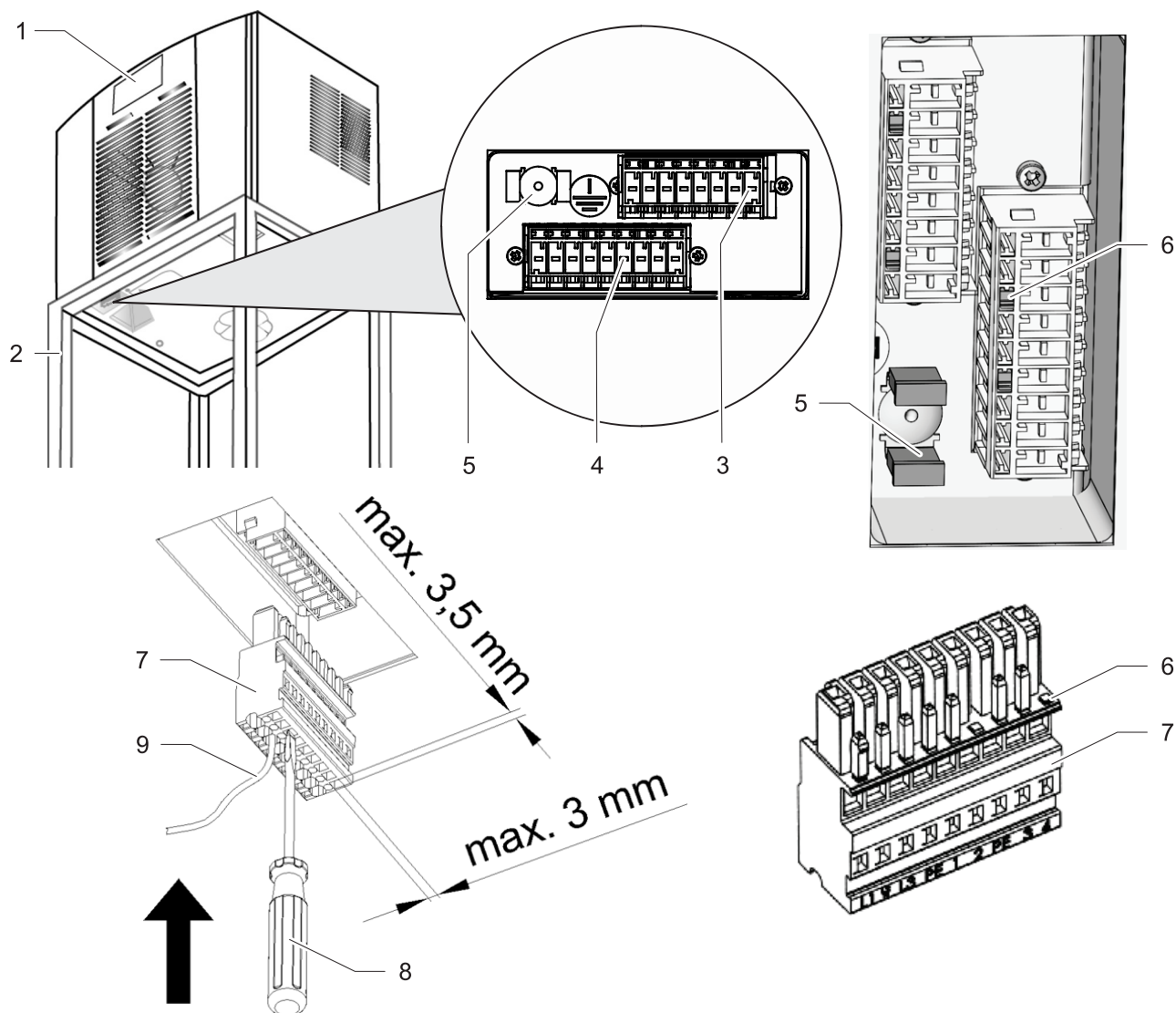
Abb. 22: Netz-Anschlussstecker Kühlgerät
