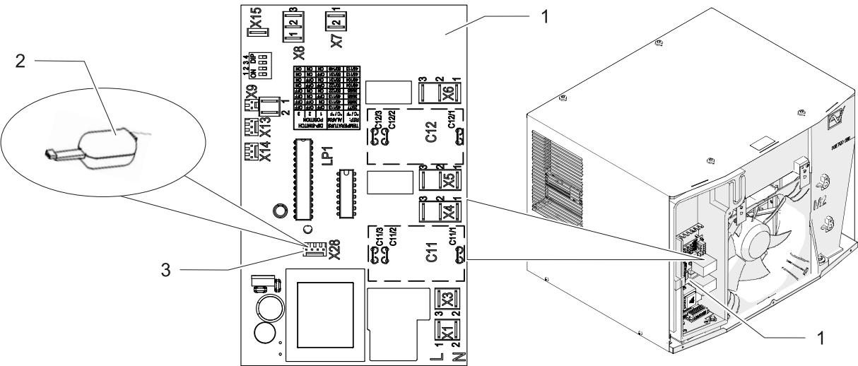
Рис. 25: Сервисный интерфейс
