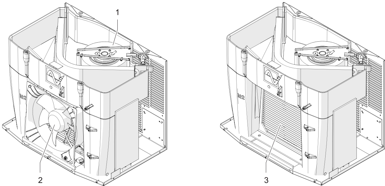
Fig. 29: Limpieza del intercambiador de calor y de los ventiladores
