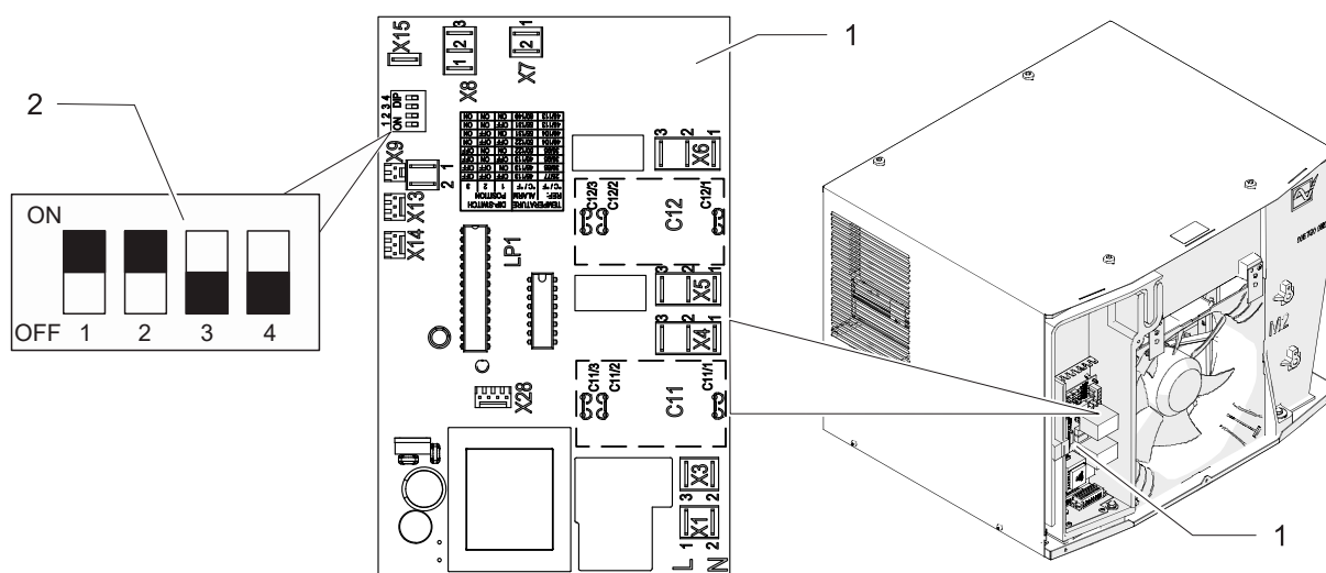
Abb. 21: DIP-Schalter einstellen
