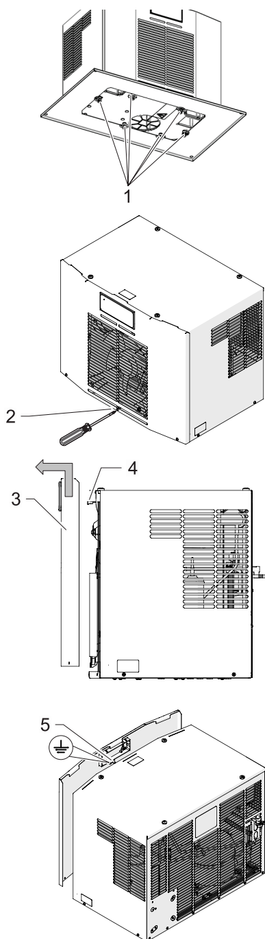
Abb. 16: Frontklappe entfernen
