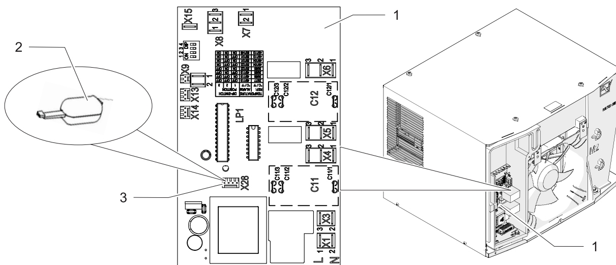
Abb. 25: Serviceschnittstelle
