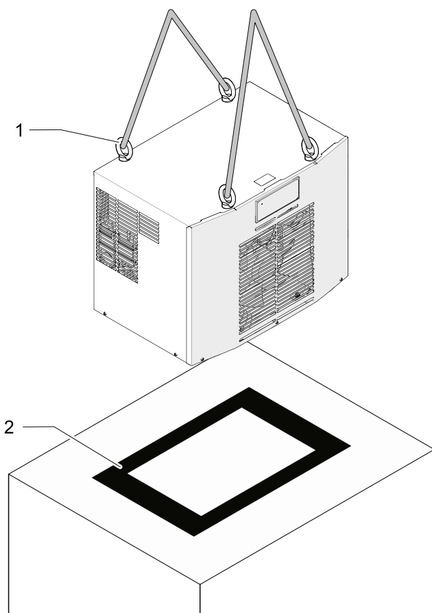
Рис. 15.: Монтаж устройства охлаждения с завертками
