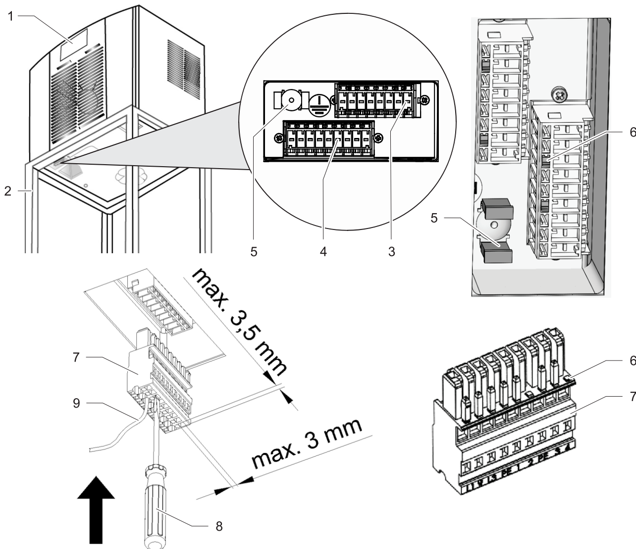
Fig. 22 : fiche de raccordement secteur du climatiseur
