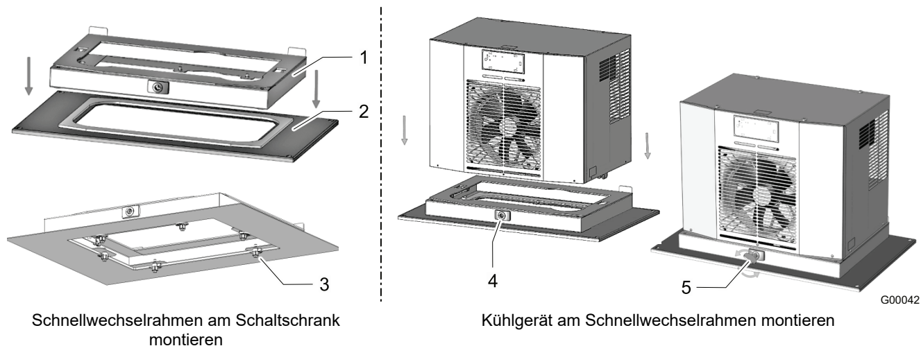
Abb. 19: Halterung montieren
