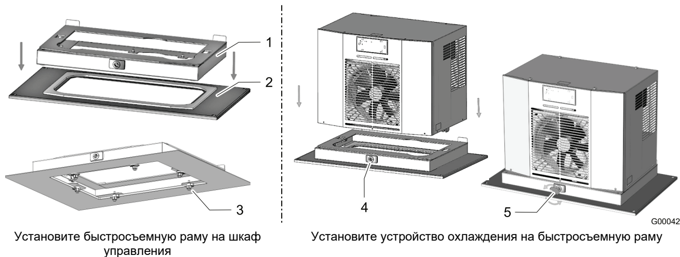
Рис. 19: Монтаж держателя
