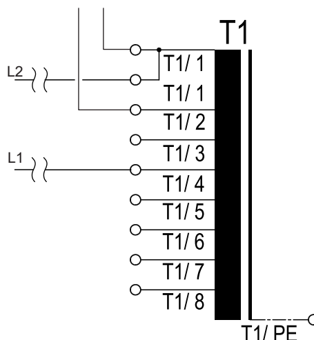
Рис. 23: Настройка сетевого напряжения на управляющем трансформаторе
