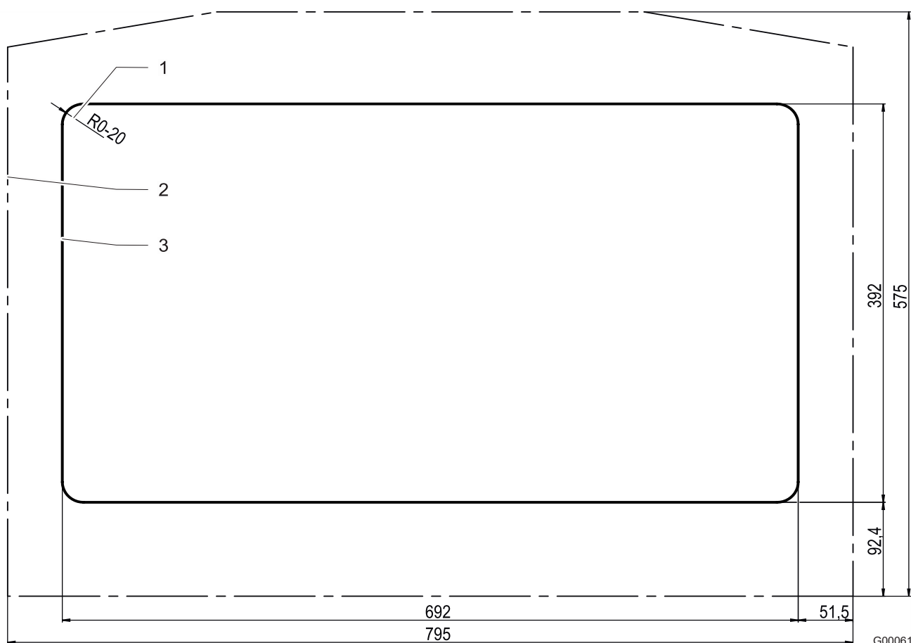
Fig. 13: Recorte del armario eléctrico
