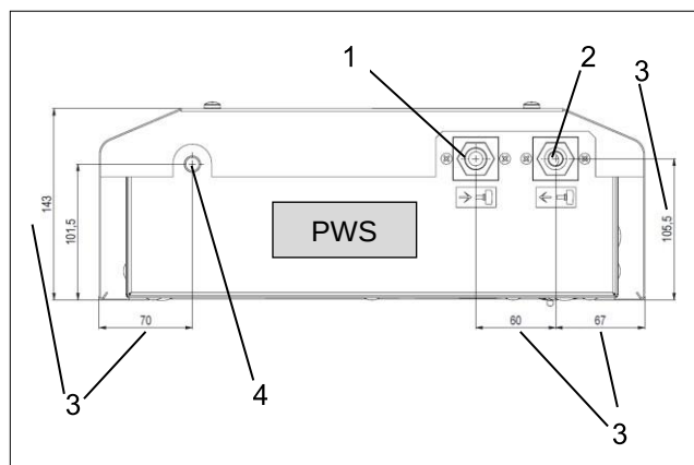
Abbildung 12 – Kühlwasseranschlüsse Wasseraustritt/-Wassereintritt
