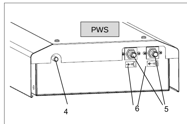
Abbildung 11 – Kühlwasseranschlüsse mit Gewinde-Schlauchtüllen
