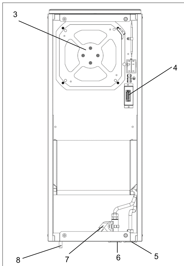
Abbildung 1 – Innenansicht Luft-/ Wasser-Wärmetauscher
