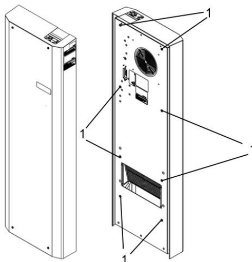
Figura 7: montar intercambiadores de calor aire/agua (colocación lateral)
