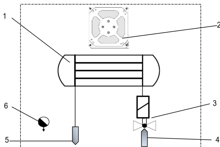
Рис. 3 - Холодильный контур
