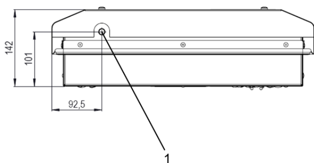
Illustration 13 – Raccordement de l'évacuation du condensat PWI
