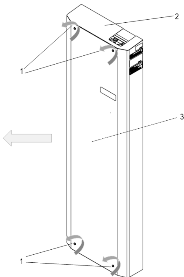
Abbildung 17 – Gerätehaube demontieren
