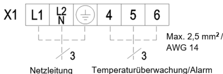
Abbildung 15 – Elektrischer Anschluss
