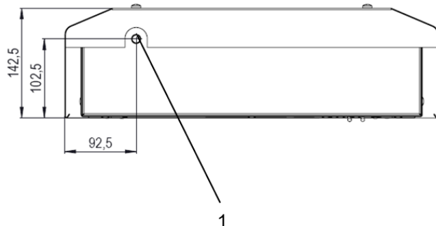
Рис. 14 – Подключение отвода конденсата PWS
