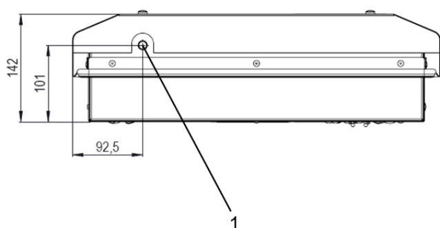
Figura 13: Toma de evacuación del condensado PWI
