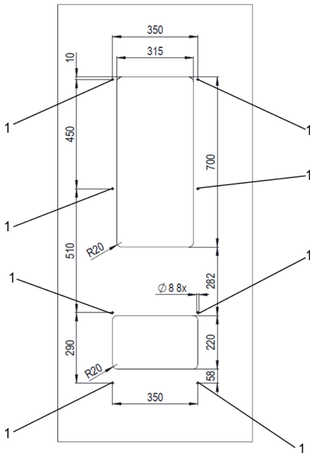
Abbildung 5 - Außenansicht Schaltschrank Bohrungen für PWS-Luft-/ Wasser-Wärmetauscher
