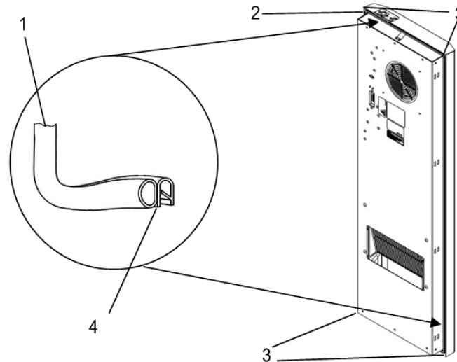
Рис. 9 - Установка профильного уплотнения Воздухо-водяной теплообменник PWI
