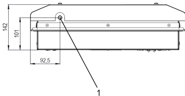
Immagine 13 – Collegamento scaricatore di condensa PWI
