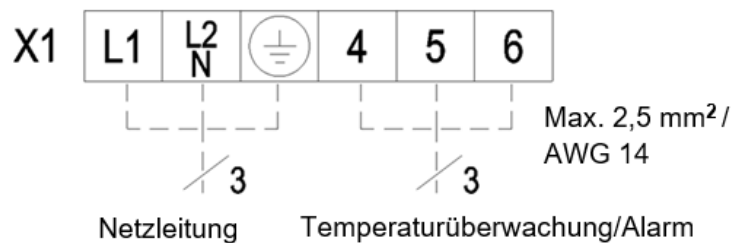
Immagine 15 – Collegamento elettrico
