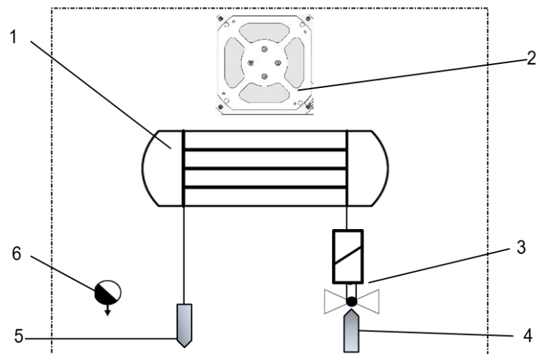
Abbildung 3 - Kältekreislauf
