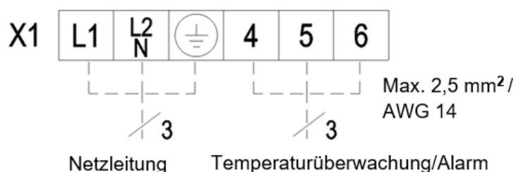
Illustration 15 – Branchement électrique
