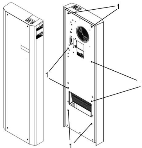
Abbildung 7 - PWS Luft-/ Wasser-Wärmetauscher (Seitenanbau) montieren
