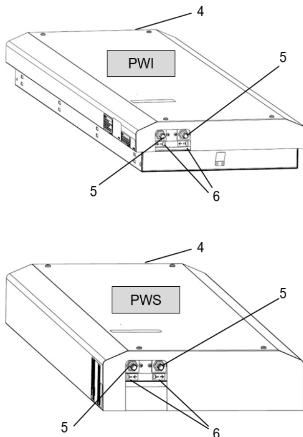
Illustration 11 – Raccordements de l'eau de refroidissement avec raccords d'extrémité filetés (vue de dessus)
