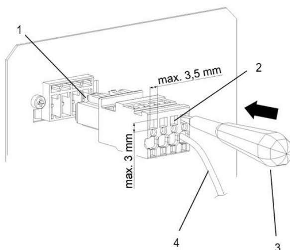
Рис. 16 - Штекерное соединение воздухо-водяного теплообменника
