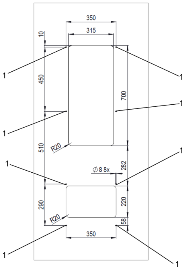
Immagine 5 – Vista interna quadro elettrico Fori per scambiatore di calore aria/acqua PWS
