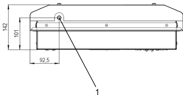
Рис. 13 – Подключение отвода конденсата PWI
