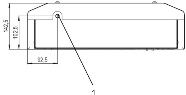
Immagine 14 – Collegamento scaricatore di condensa PWS
