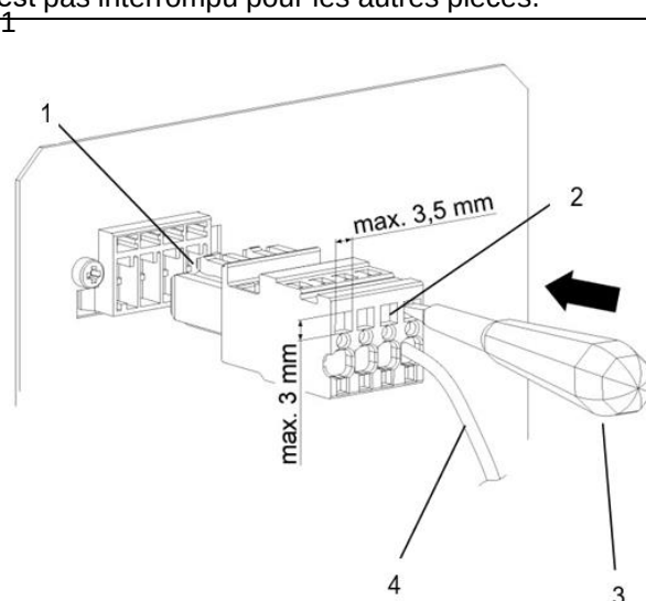
Illustration 16 - Connexion de l'échangeur thermique air/eau au réseau
