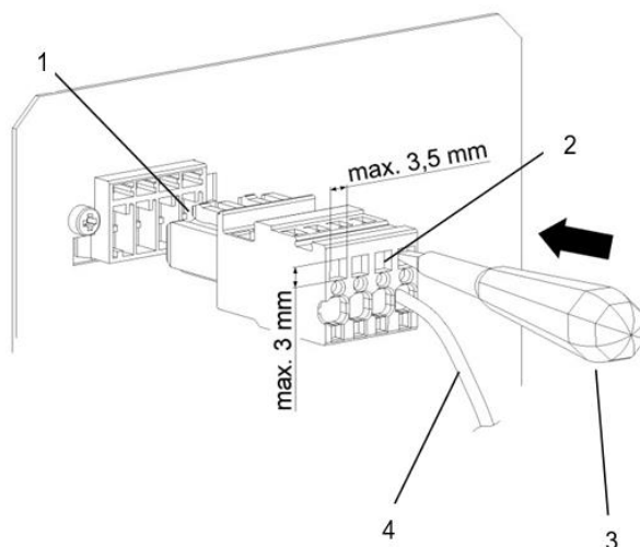
Abbildung 16 - Steckerverbindung Luft-/ Wasser-Wärmetauscher
