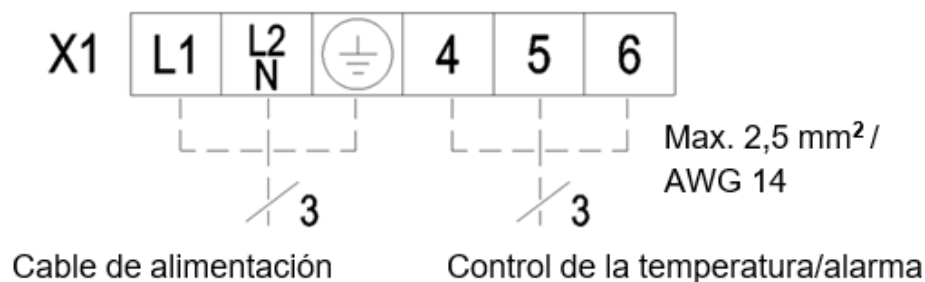
Figura 15 – Conexión eléctrica
