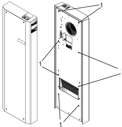
Рис. 7 - Монтаж воздухо-водяного теплообменника PWS (боковая навеска)
