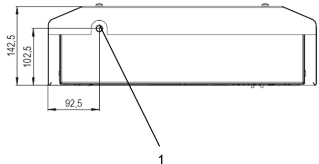
Abbildung 14 – Anschluss Kondensatablauf PWS
