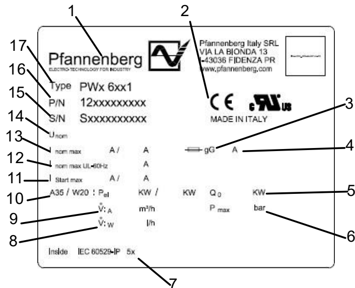
Abbildung 4 - Typenschild EU-Mitgliedsländer
