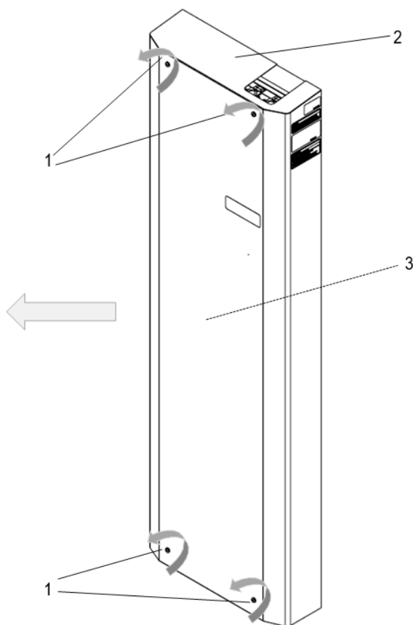
Illustration 17 – Démontage du capot de l'appareil
