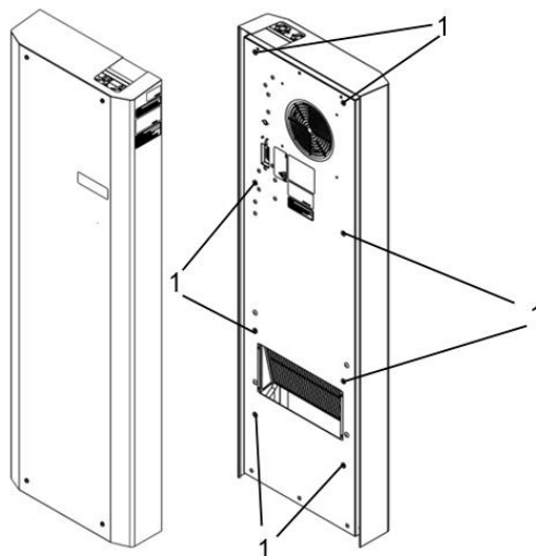
Illustration 7 - Monter l'échangeur thermique air/eau PWS (montage latéral)
