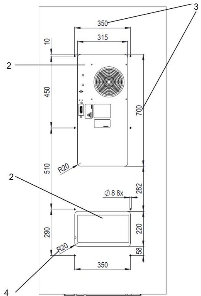
Abbildung 6 - Außenansicht Schaltschrank Ausschnitt für PWS-Luft-/ Wasser-Wärmetauscher
