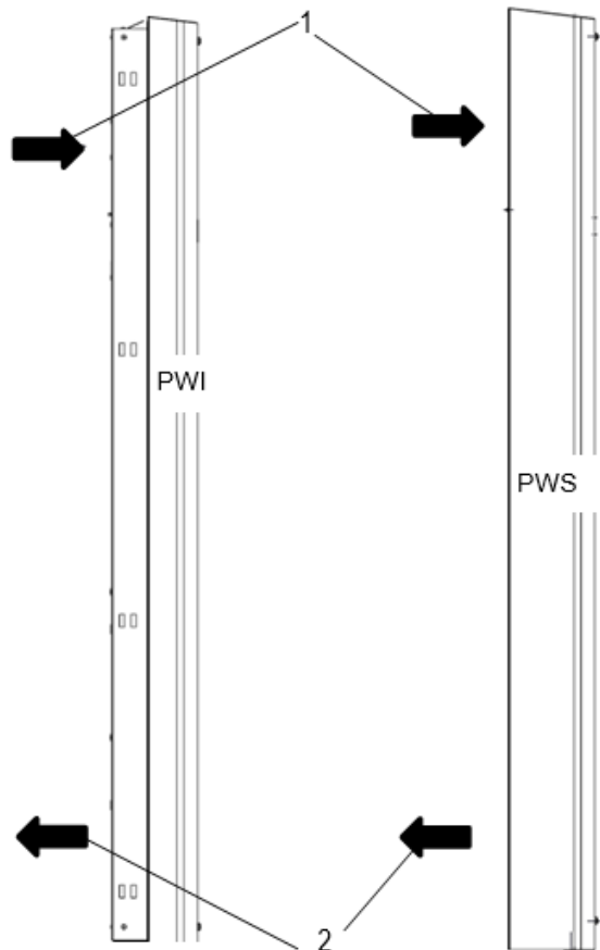
Abbildung 1 - Seitenansicht Luftstromprinzip PWI/PWS-Luft-/ Wasser-Wärmetauscher
